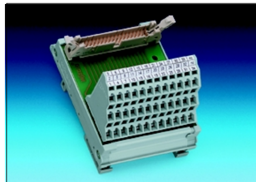
Kleiner und feiner: Überarbeitete WAGO Übergabemodule für Flachbandkabel.
