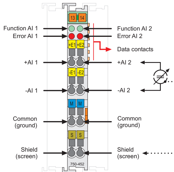
Fig. 2.1.1-1: 2-Channel Analog Input Module 750-452
