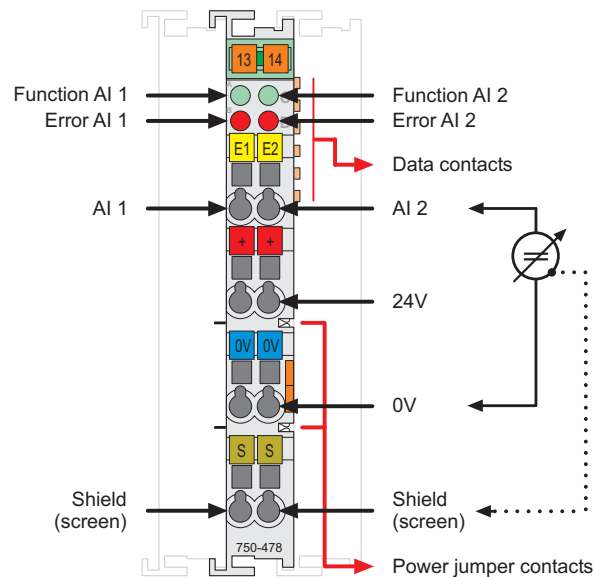
Fig. 2.1.1-1: 2-Channel Analog Input Module 750-478
