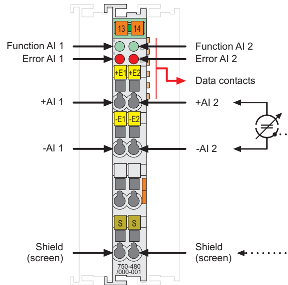
Fig. 2.1.2-1: 2-Channel Analog Input Module 0-20 mA
