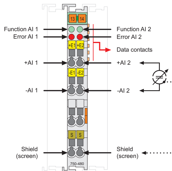
Fig. 2.1.1-1: 2-Channel Analog Input Module 0-20 mA
