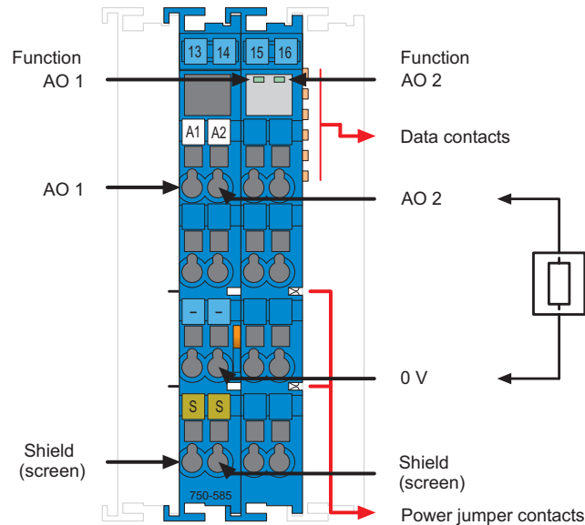
Fig. 2.1.1-1: 2-Channel Analog Output Module 750-585
