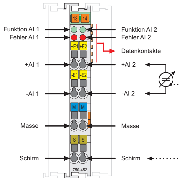
Abb. 2.1.1-1: 2-Kanal Analog Eingangsklemme 750-452
