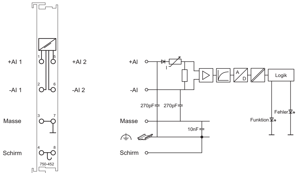
Abb. 2.1.1-3: 2-Kanal Analog Eingangsklemme 750-452
