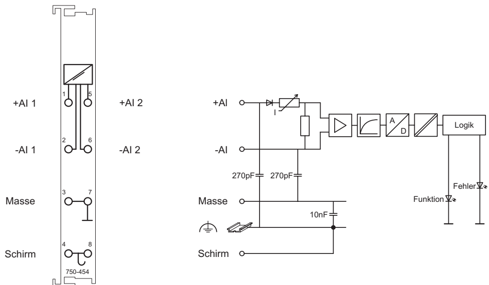
Abb. 2.1.1-3: 2-Kanal Analog Eingangsklemme 750-454
