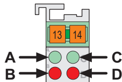
Abb. 2.1.1-2: Anzeigeelemente g045202x
