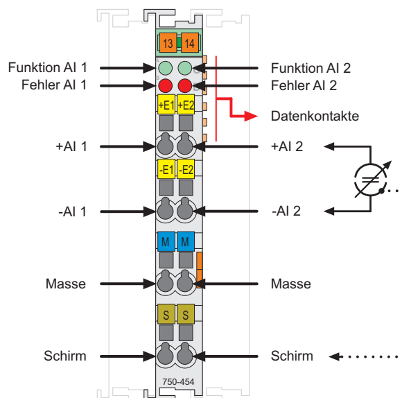
Abb. 2.1.1-1: 2-Kanal Analog Eingangsklemme 750-454
