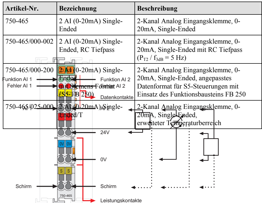
Abb. 2.1.1-1: Ansicht
