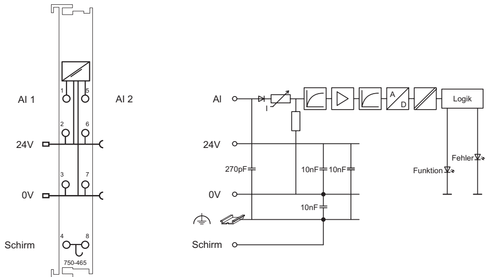
Abb. 2.1.1-3: Schematisches Schaltbild
