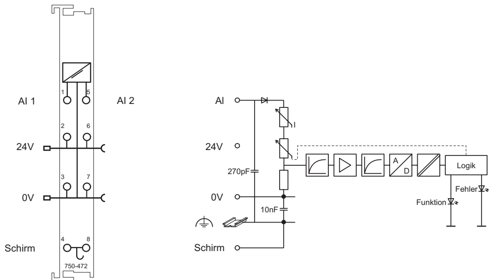
Abb. 2.1.1-3: 2-Kanal Analog Eingangsklemme 750-472
