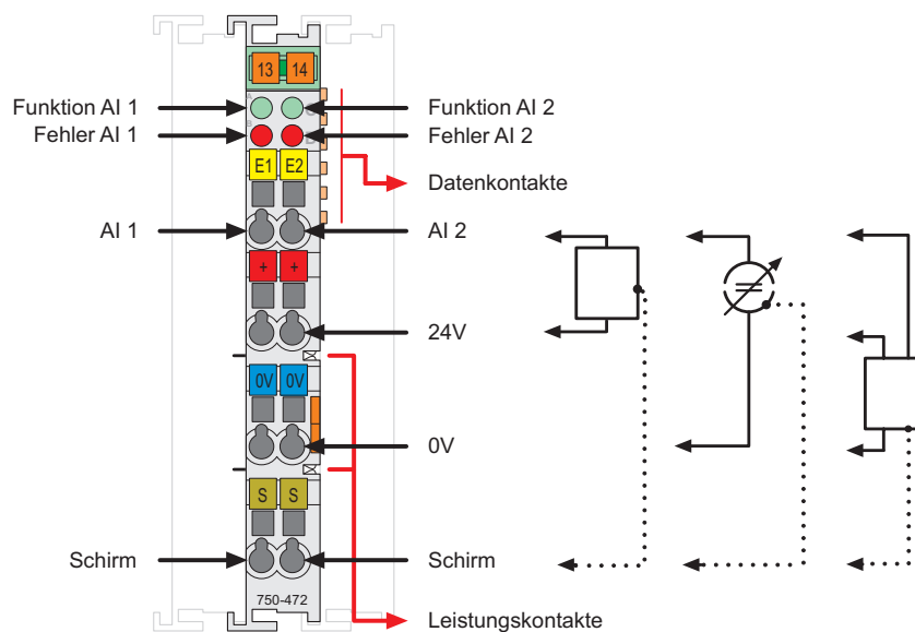
Abb. 2.1.1-1: 2-Kanal Analog Eingangsklemme 750-472
