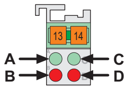
Abb. 2.1.1-2: Anzeigeelemente g045202x
