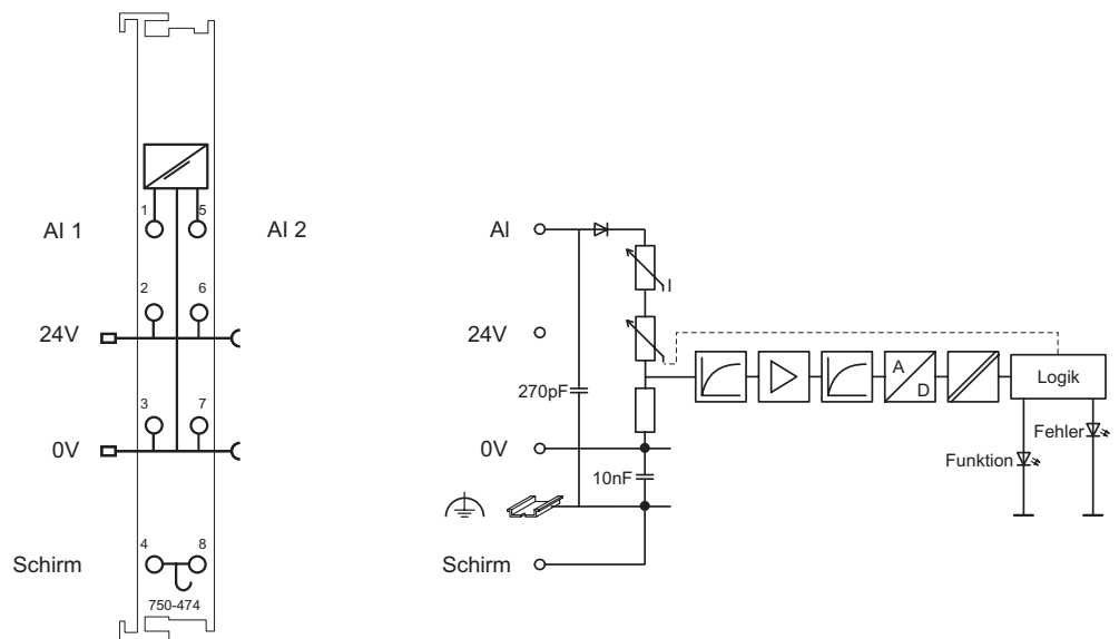
Abb. 2.1.1-3: Schematisches Schaltbild
