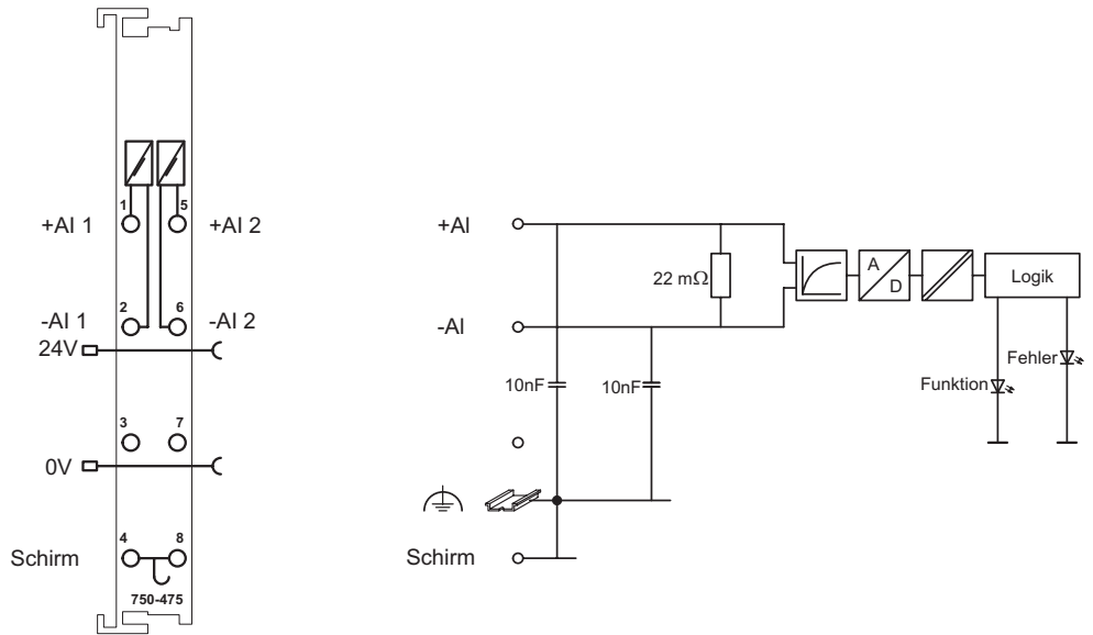
Abb. 2.1.1-3: Schematisches Schaltbild
