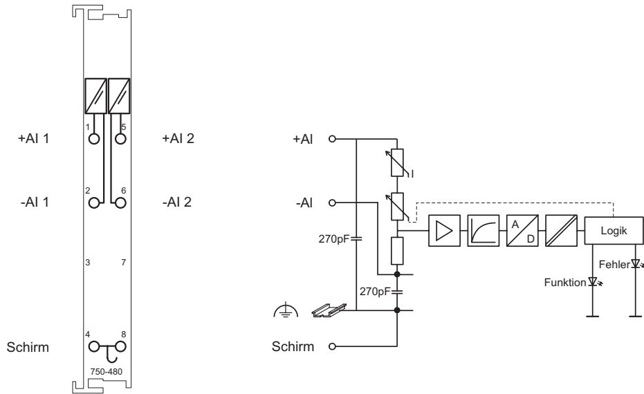
Abb. 2.1.2-3: 2-Kanal Analog Eingangsklemme 0-20 mA
