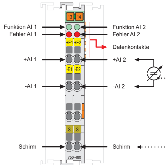
Abb. 2.1.2-1: 2-Kanal Analog Eingangsklemme 0-20 mA
