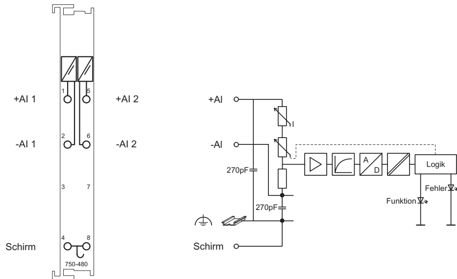
Abb. 2.1.1-3: 2-Kanal Analog Eingangsklemme 0-20 mA
