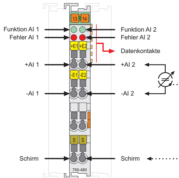
Abb. 2.1.1-1: 2-Kanal Analog Eingangsklemme 0-20 mA
