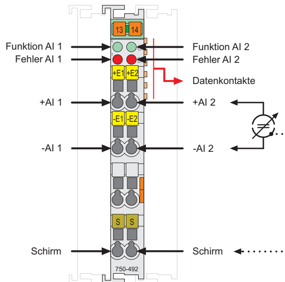
Abb. 1.1.1-1: 2-Kanal Analog Eingangsklemme 4-20 mA
