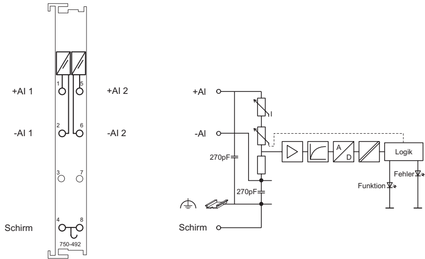
Abb. 1.1.1-3: 2-Kanal Analog Eingangsklemme 4-20 mA
