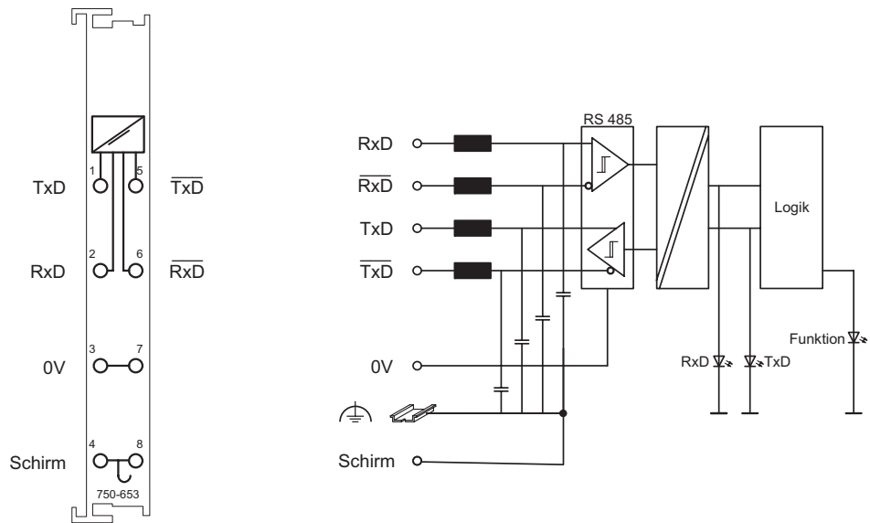
Abb. 2.1.1-3: Serielle Schnittstelle 750-653
