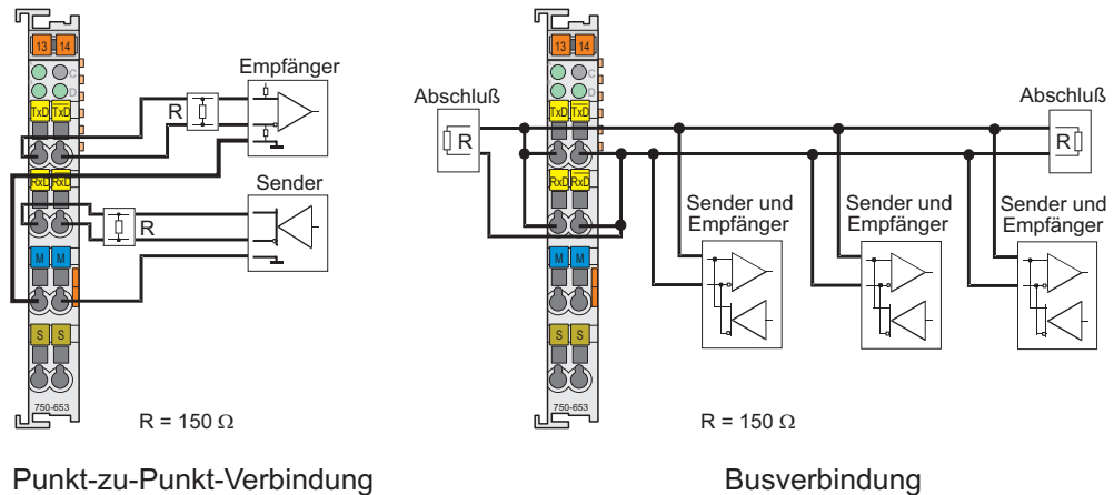
Abb. 2.1.1-4: Einsatz der RS 485 Schnittstellenklemme
