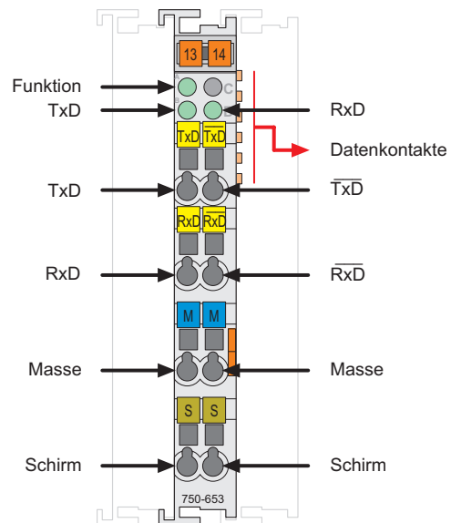
Abb. 2.1.1-1: Serielle Schnittstelle 750-653
