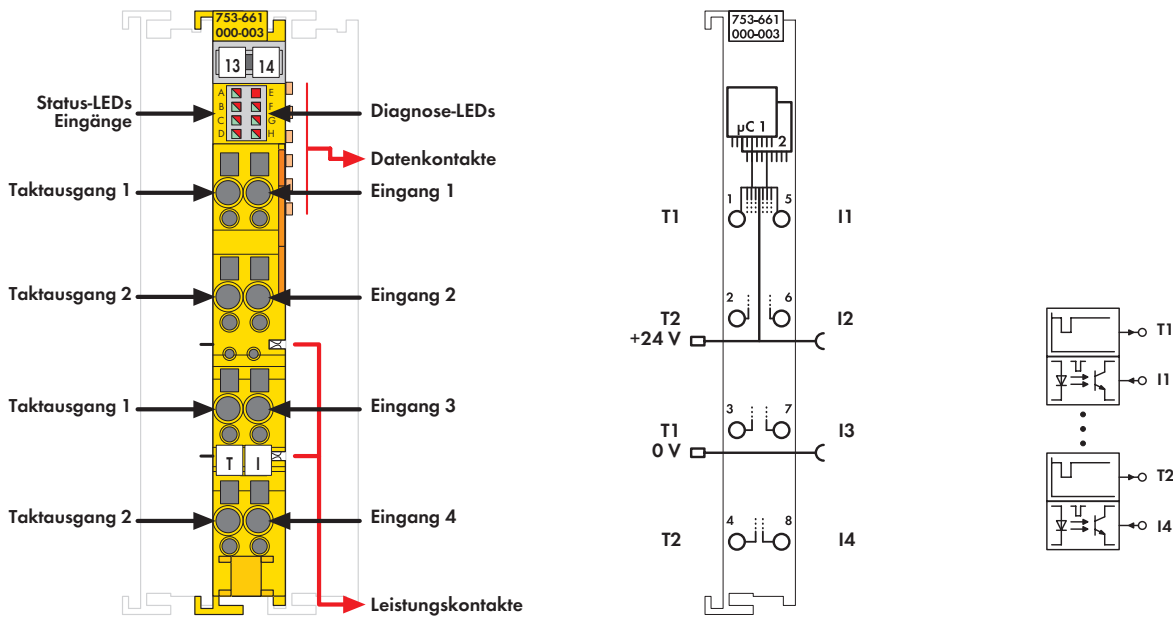
Abb. Serie 753 / Lieferung ohne Mini-WSB
