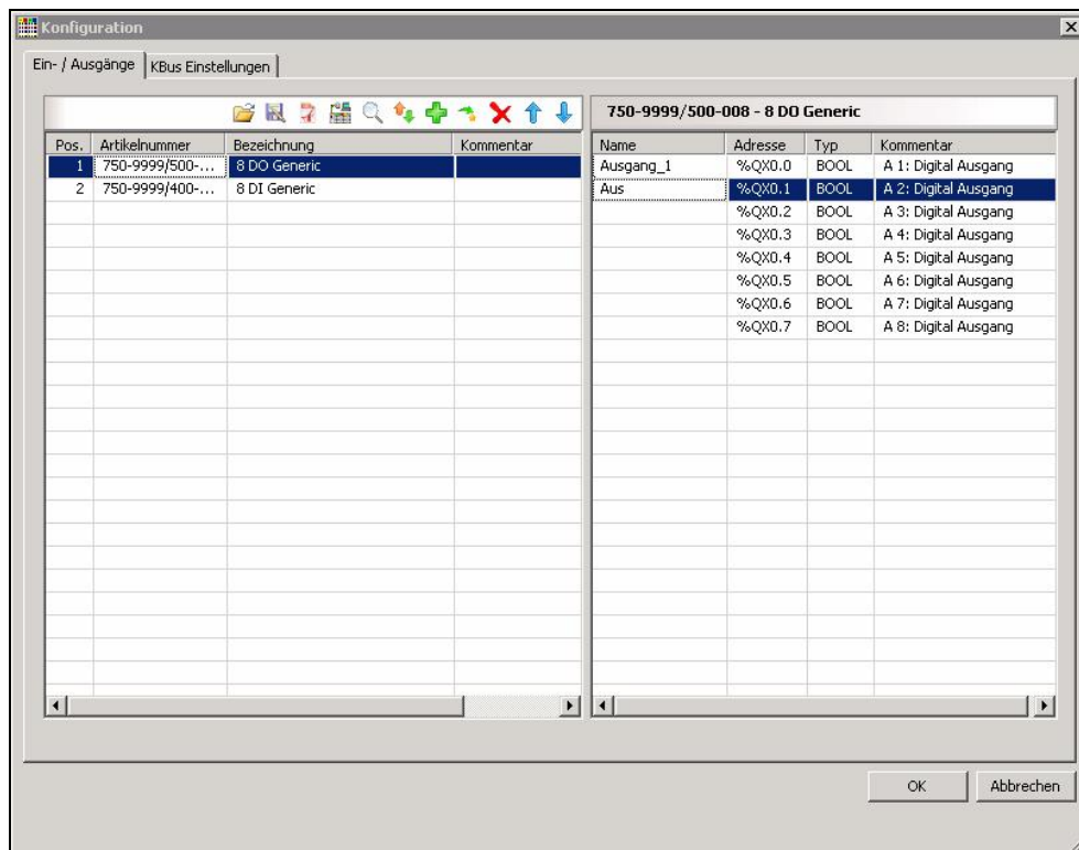
Abbildung 47: Variablendeklaration
