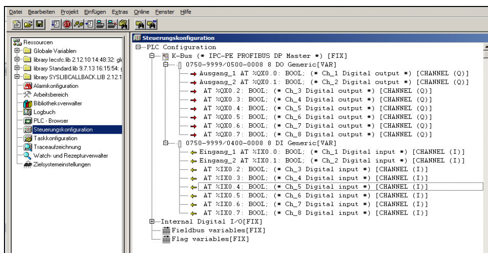
Abbildung 48: Steuerungskonfiguration: Busklemmen mit den dazugehörigen Adressen
