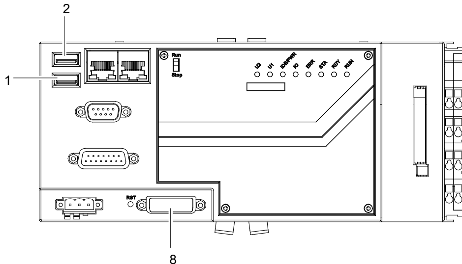
Abbildung 86: DVI-I-Schnittstelle X7 und USB-Schnittstellen X10/11
