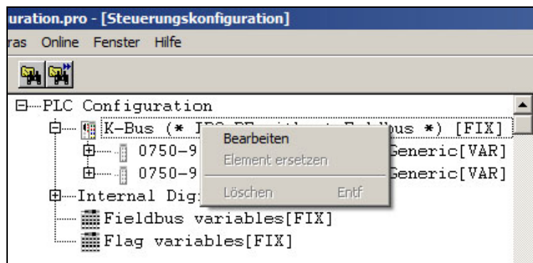
Abbildung 42: Steuerungskonfiguration: Bearbeiten
