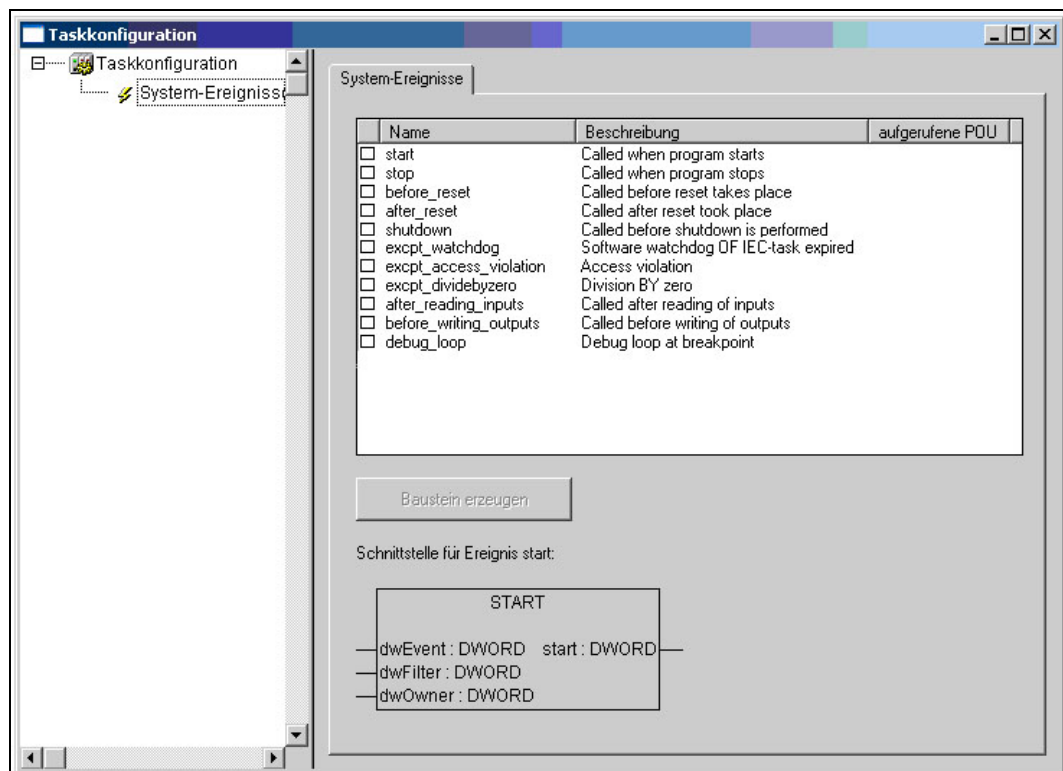
Abbildung 62: Systemereignisse
