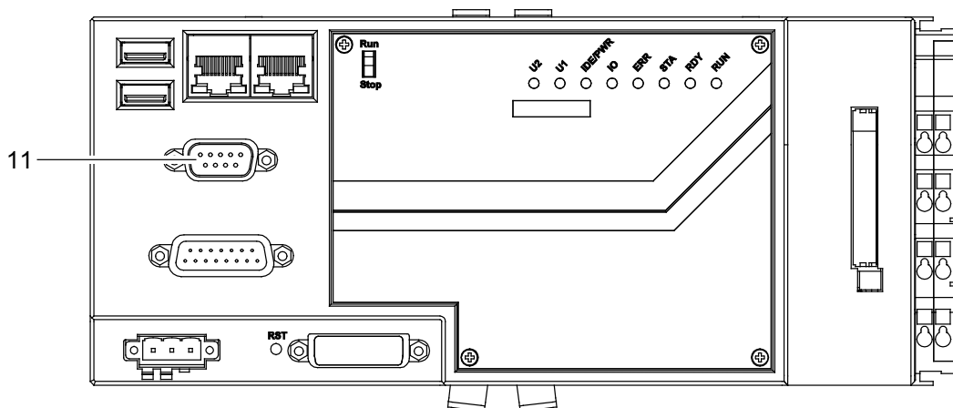
Abbildung 85: RS-232-Schnittstelle X6
