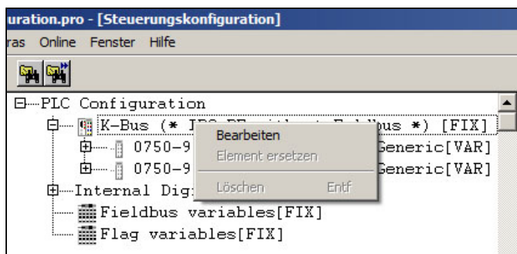
Abbildung 43: Steuerungskonfiguration: Bearbeiten
