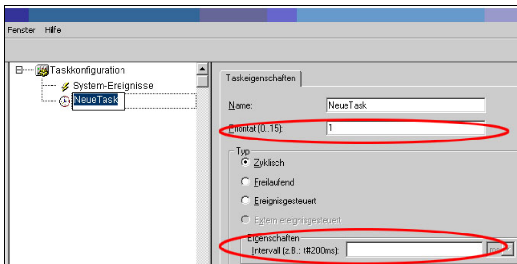
Abbildung 61: Task-Namen ändern 2
