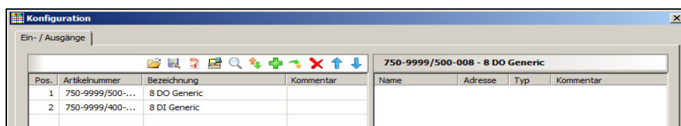
Abbildung 44: Konfiguration
