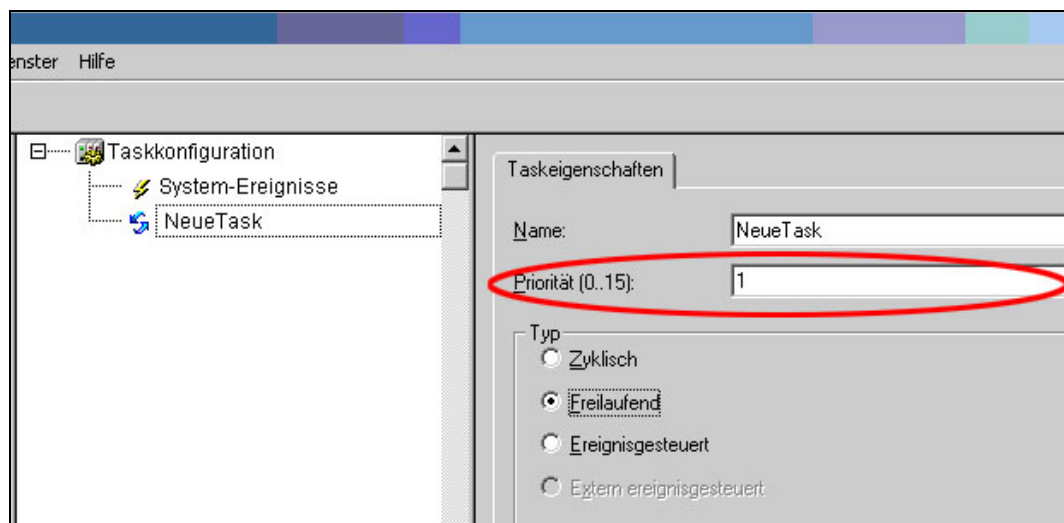
Abbildung 62: Freilaufende Tasks
