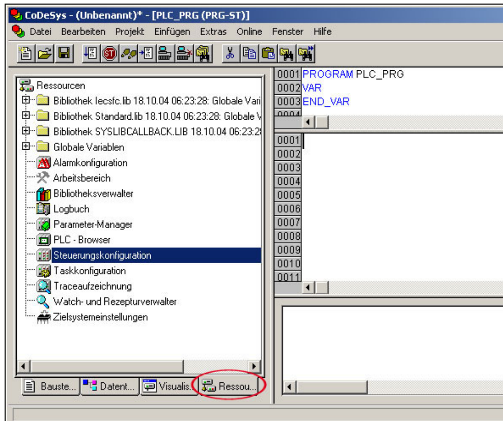
Abbildung 89: Karteireiter „Ressourcen“
