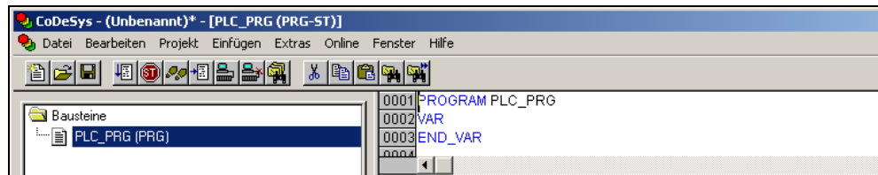
Abbildung 86: PLC_PRG
