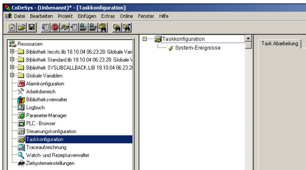
Abbildung 58: Task-Konfiguration
