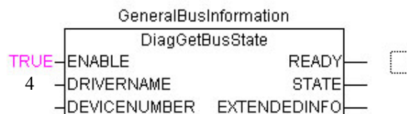
Abbildung 92: Instanz des Funktionsbausteins DiagGetBusState() in FUP
