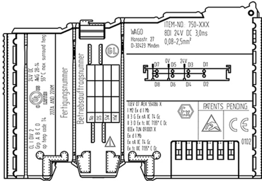
Abbildung 128: Beispiel für die seitliche Bedruckung der ATEX- und IECEx-zugelassenen Busklemmen.
