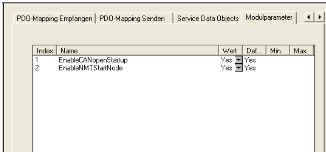
Abbildung 84: Karteireiter „Modulparameter“
