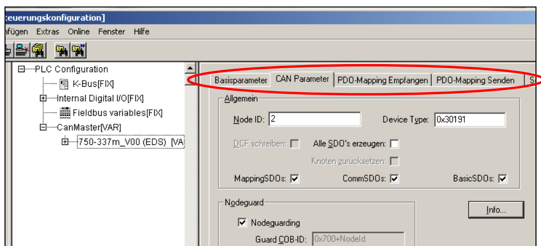
Abbildung 74: Node-ID einstellen
