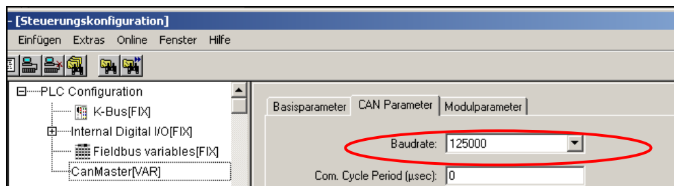
Abbildung 100: Baudrate einstellen
