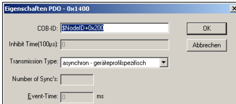
Abbildung 82: PDO-Eigenschaften-Fenster
