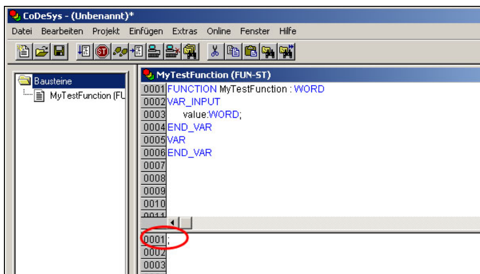
Abbildung 109: Fenster „MyTestFunction“
