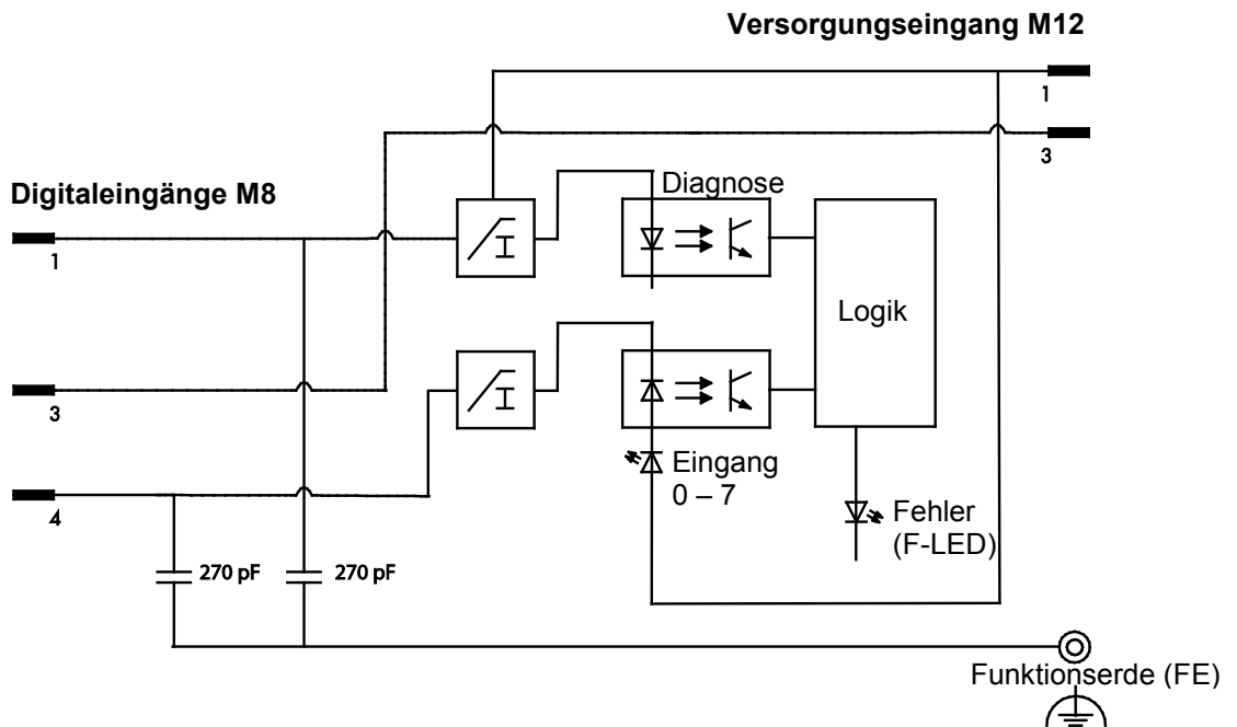
Abbildung 6: Schematisches Schaltbild
