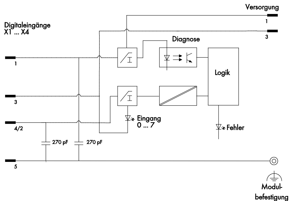
Abbildung 6: Schematisches Schaltbild
