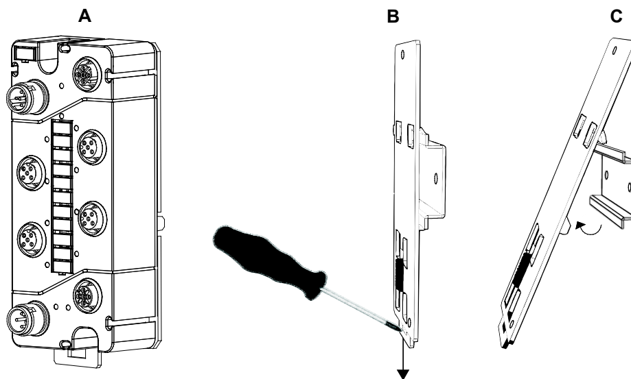
Abbildung 21: Modul mit Tragschienenadapter von der Tragschiene entfernen
