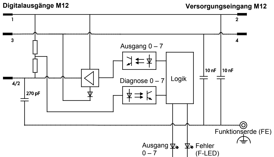
Abbildung 6: Schematisches Schaltbild
