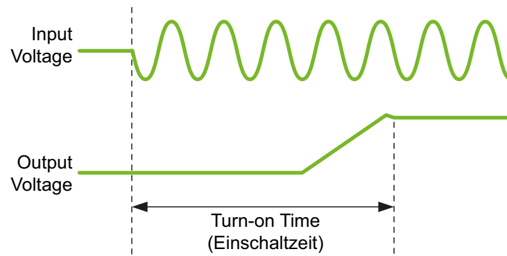
Abbildung 11: Einschaltzeit
