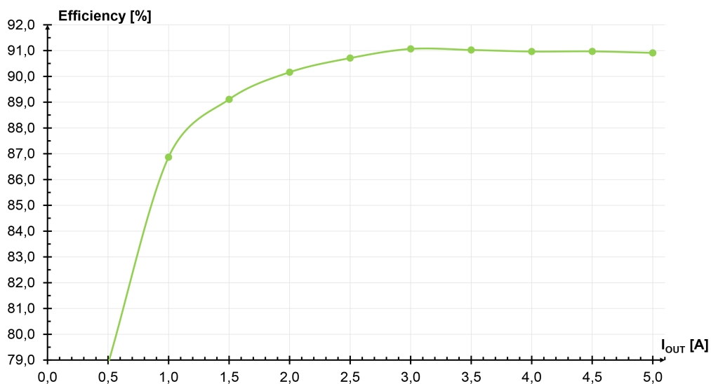
Abbildung 7: Wirkungsgrad bei AC 230 V
