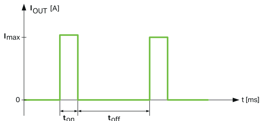
Abbildung 10: Hiccup-Mode
