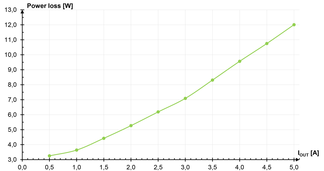
Abbildung 8: Verlustleistung bei AC 230 V
