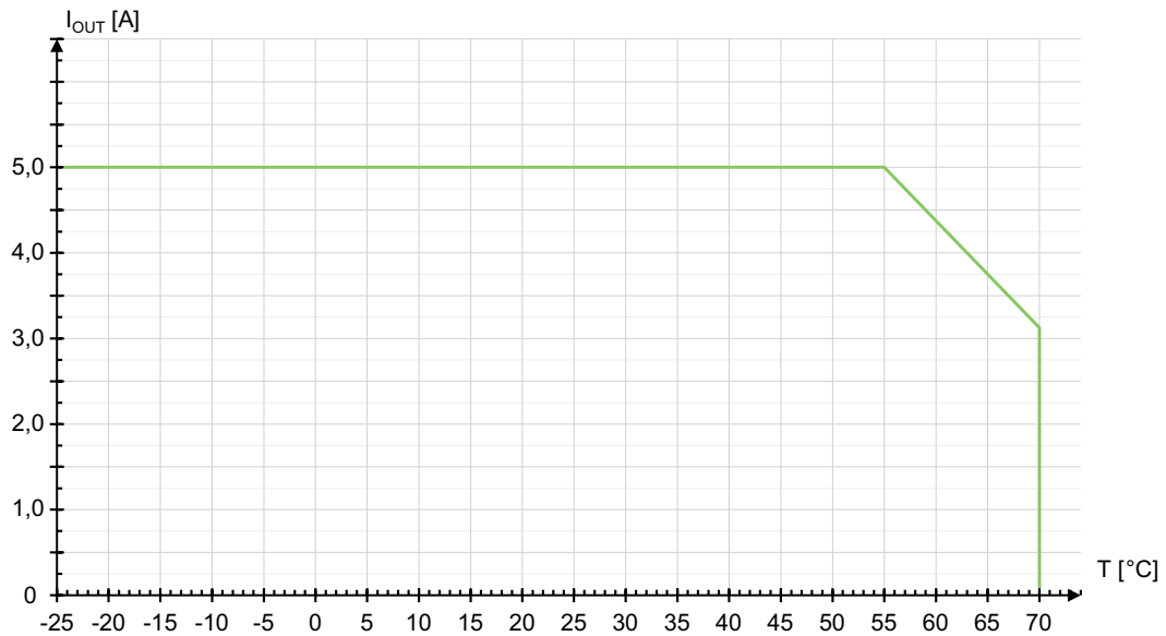
Abbildung 9: Derating (temperaturabhängig)
