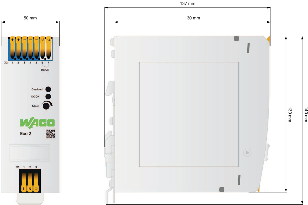
Abbildung 7: Abmessungen
