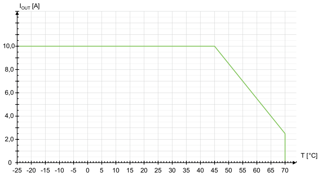
Abbildung 10: Derating (temperaturabhängig)
