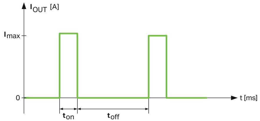
Abbildung 11: Hiccup-Mode
