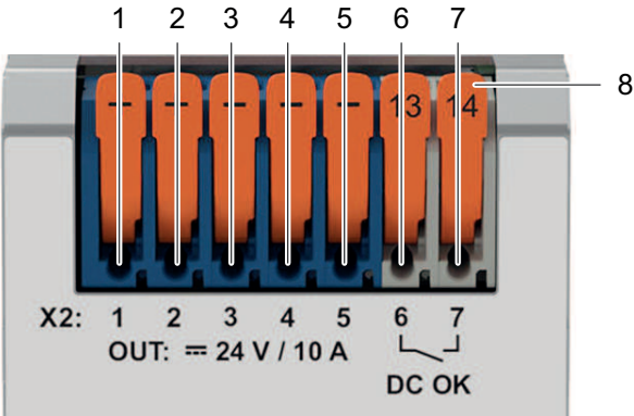
Abbildung 4: Anschluss Ausgang X2
