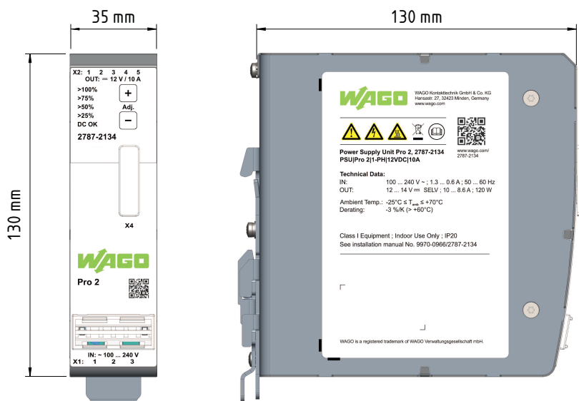
Ilustracja 9: Wymiary
