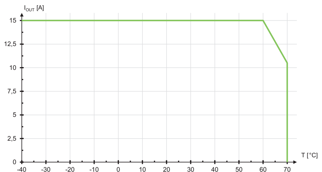
Ilustracja 37: Ograniczenie obciążenia (w zależności od temperatury)
