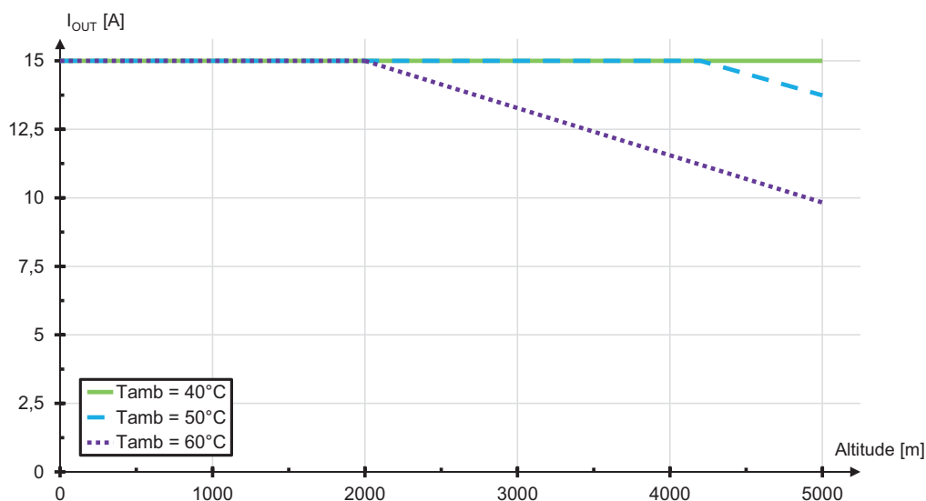
Ilustracja 38: Ograniczenie obciążenia (w zależności od lokalizacji)
