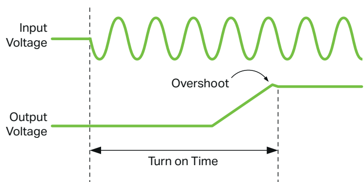
Ilustracja 10: Czas załączania
