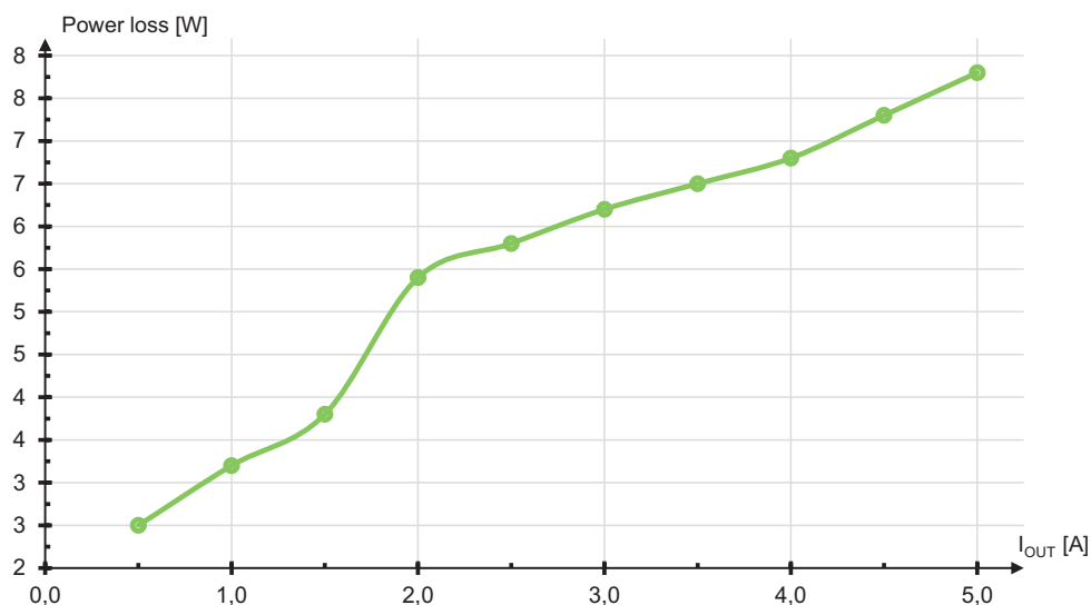
Ilustracja 12: Moc strat (typ.) przy 230 V AC
