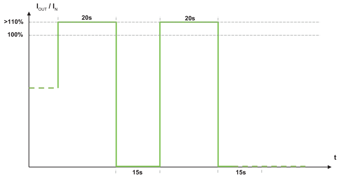
Ilustracja 39: Tryb „Constant current“
