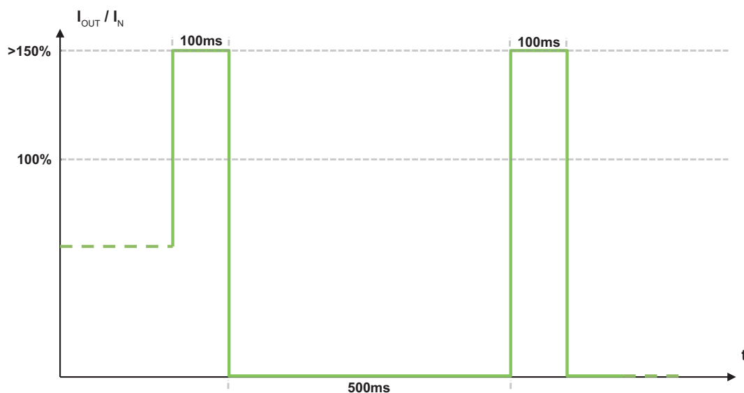
Ilustracja 41: Tryb „Hiccup”
