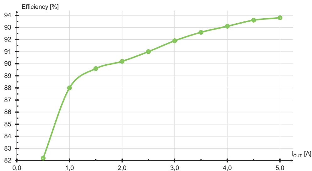
Ilustracja 11: Sprawność (typ.) przy 230 V AC
