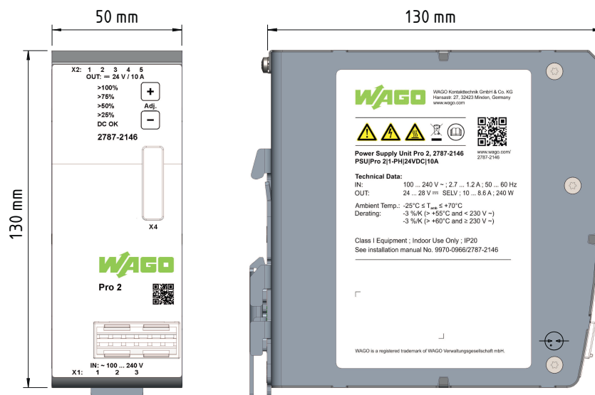
Ilustracja 9: Wymiary
