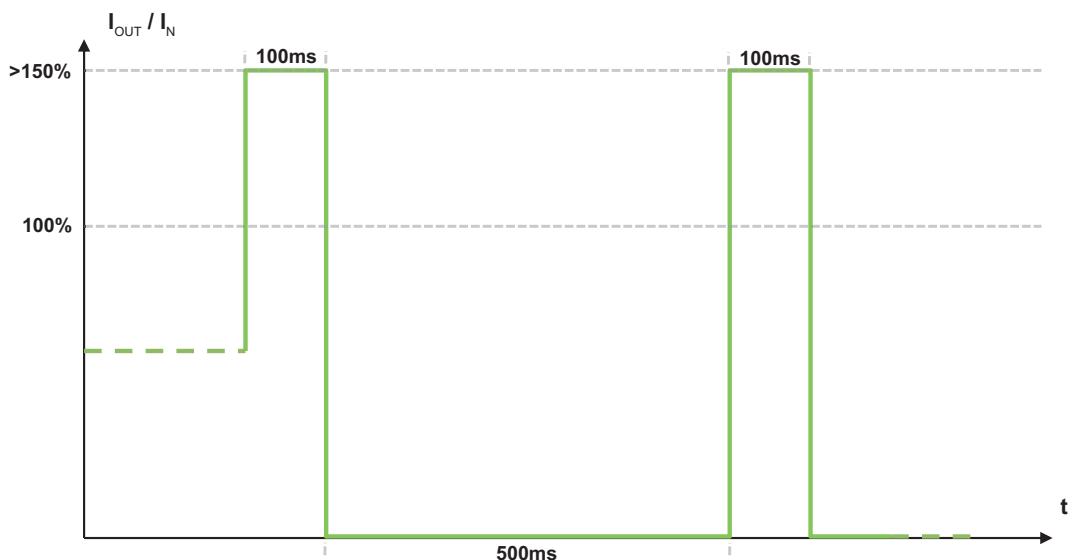
Ilustracja 41: Tryb „Hiccup“
