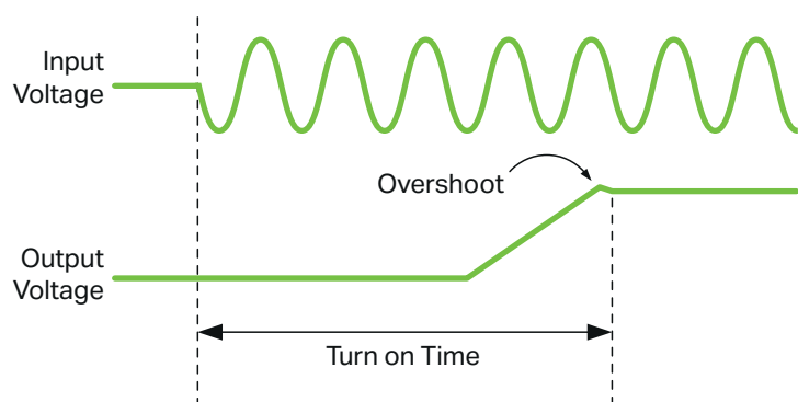
Ilustracja 10: Czas załączania
