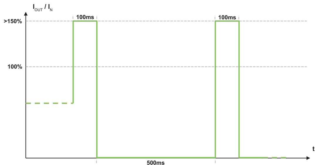
Ilustracja 41: Tryb „Hiccup“
