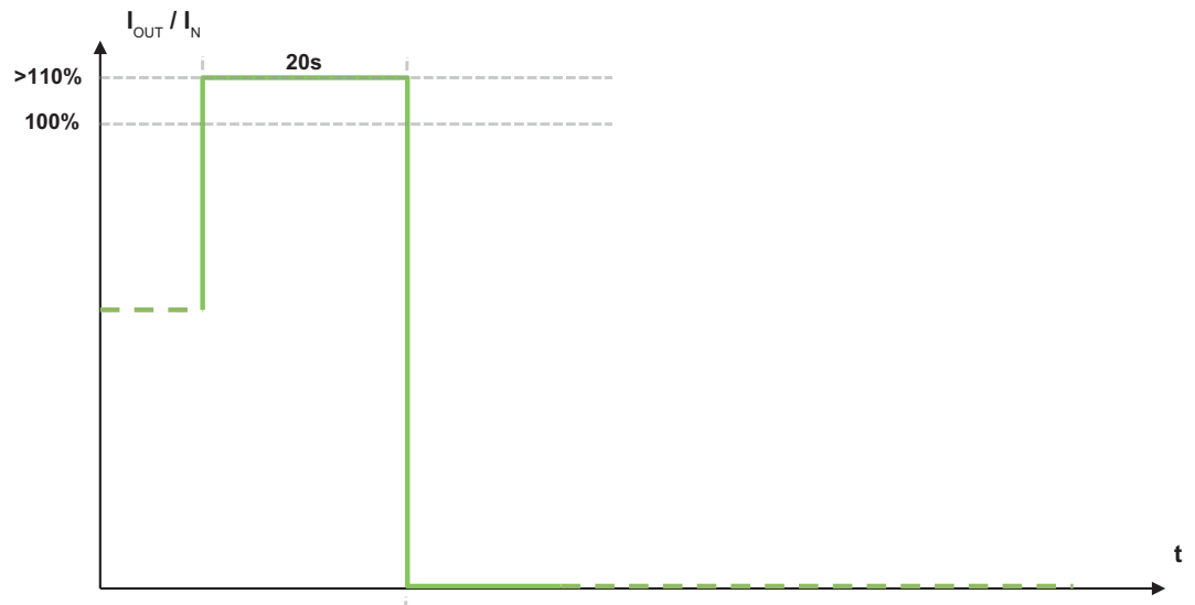
Ilustracja 40: Tryb „Constant current (latching mode)“
