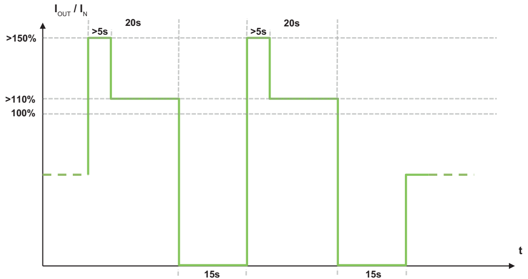
Ilustracja 43: Tryb „PowerBoost” w połączeniu z trybem „Constant current”
