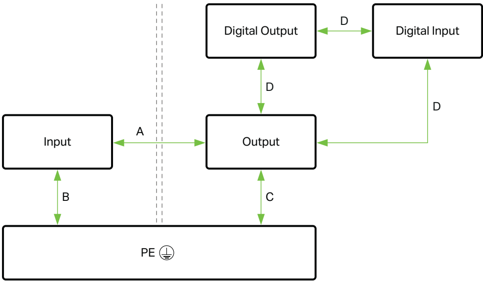
Ilustracja 13: Wytrzymałość napięciowa
