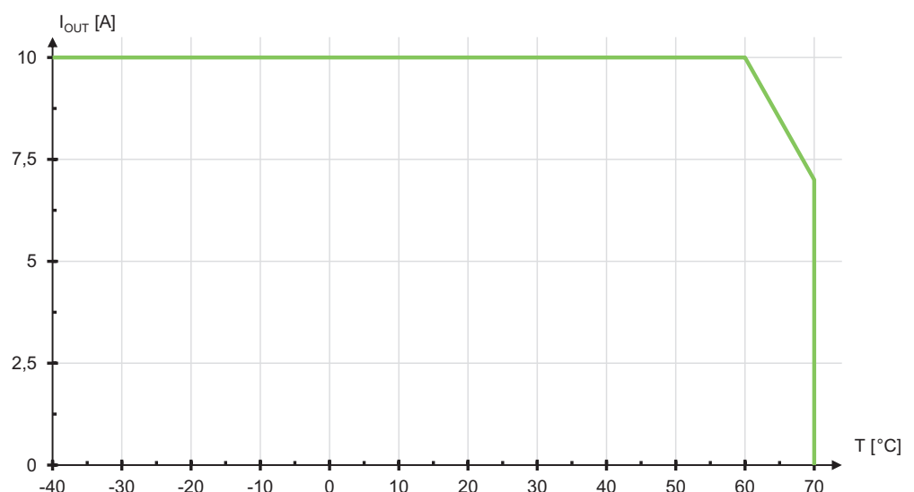
Ilustracja 37: Ograniczenie obciążenia (w zależności od temperatury)
