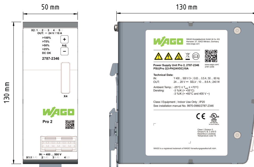
Ilustracja 9: Wymiary
