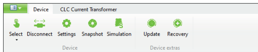
Ilustracja 24: Zakładka „Device“
