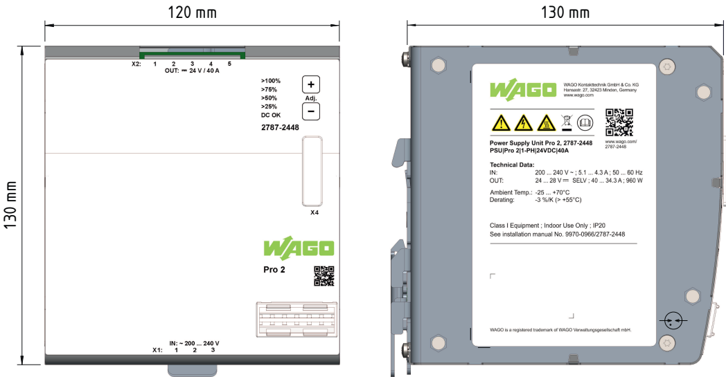
Ilustracja 9: Wymiary
