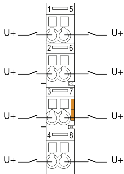
Abbildung 6: Beispiel 1-Leiter-Anschluss
