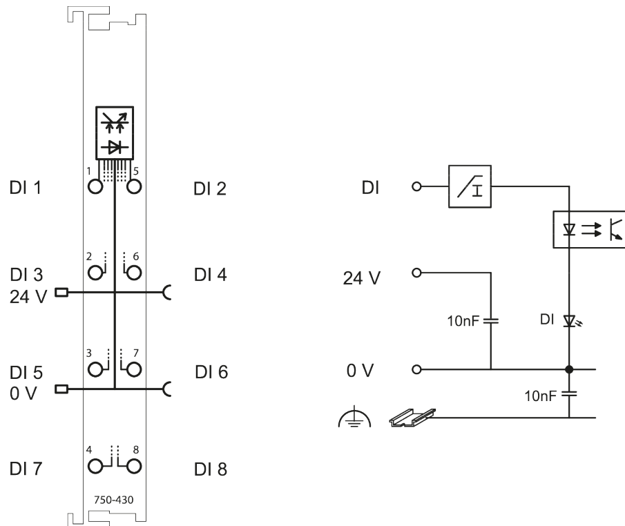
Abbildung 5: Schematisches Schaltbild
