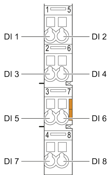
Abbildung 3: CAGE CLAMP®-Anschlüsse
