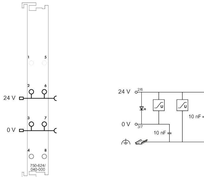
Abbildung 5: Schematisches Schaltbild
