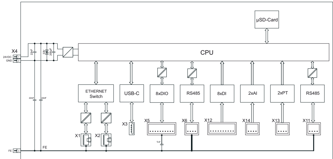
Abbildung 7: Schematisches Schaltbild
