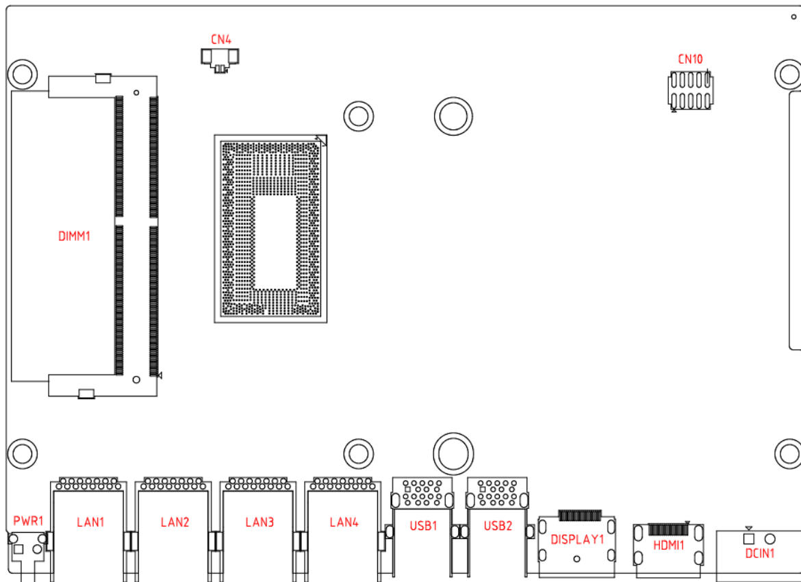
Abbildung 3: Schematisches Schaltbild – CPU-/Memory-Seite
