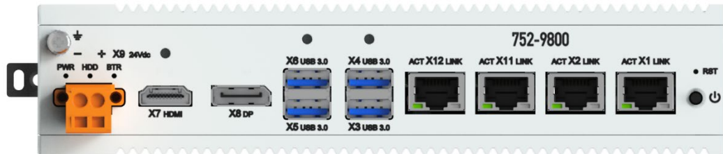
Abbildung 1: Ansicht Vorderseite
