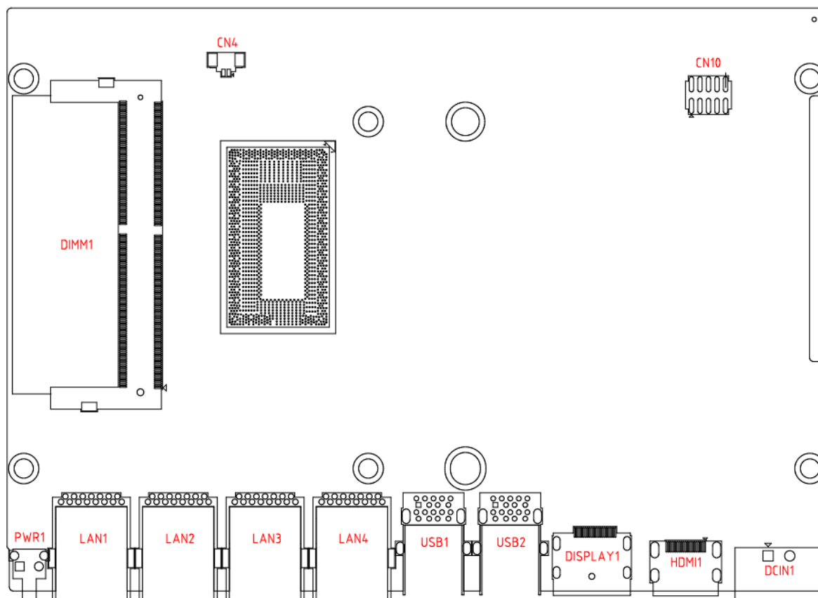
Ilustracja 3: Schemat połączeń wewnętrznych – strona CPU/pamięć
