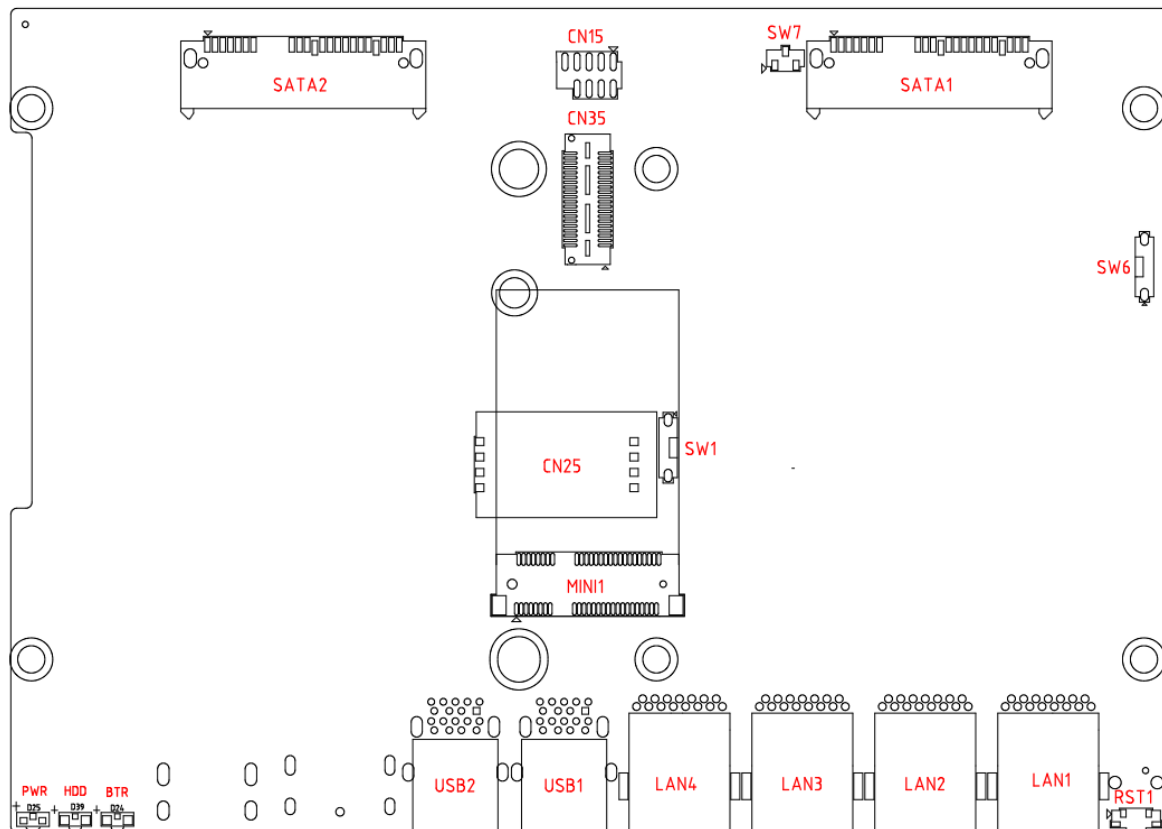
Ilustracja 4: Schemat połączeń wewnętrznych – strona SATA/mPCIe
