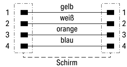
Pin 1 ... 4: 0,34 mm 2
