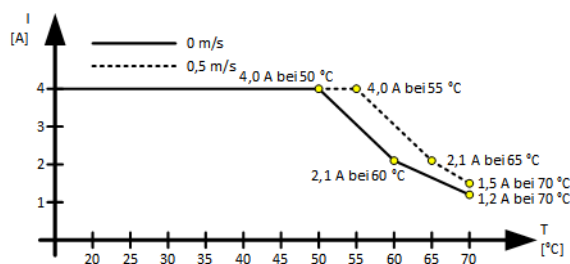
Abbildung 5: Derating 765-1701/200-000
