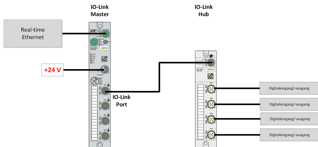
Abbildung 7: Anschlussbeispiel eines IO-Link-Hubs 765-1701/200-000 an einen IO-Link-Master
