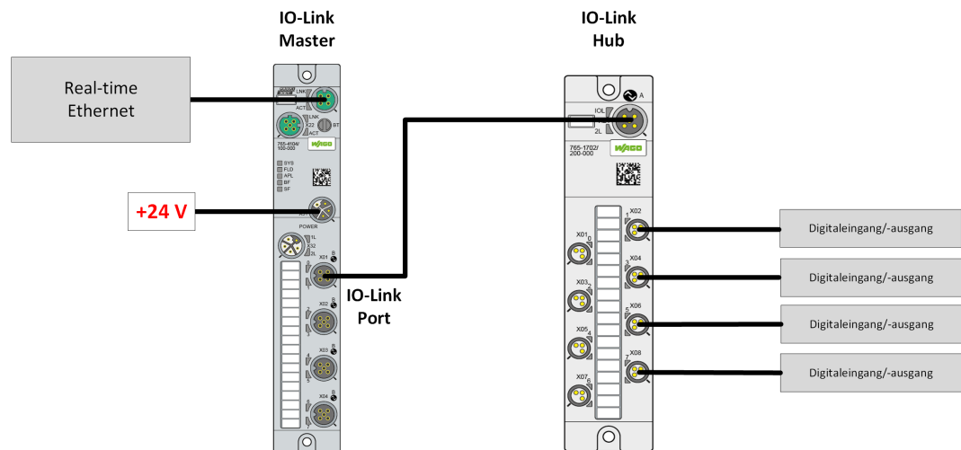
Abbildung 7: Anschlussbeispiel eines IO-Link-Hubs 765-1702/200-000 an einen IO-Link-Master
