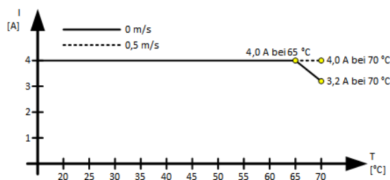
Abbildung 5: Derating 765-1702/200-000
