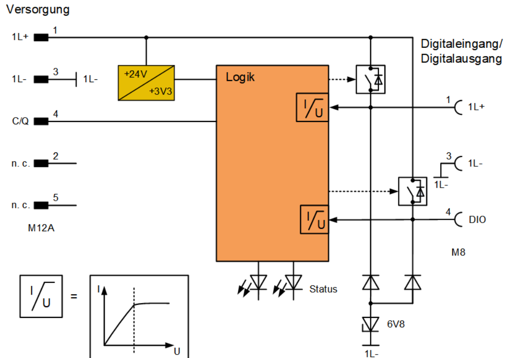
Abbildung 4: Schematisches Schaltbild je Port
