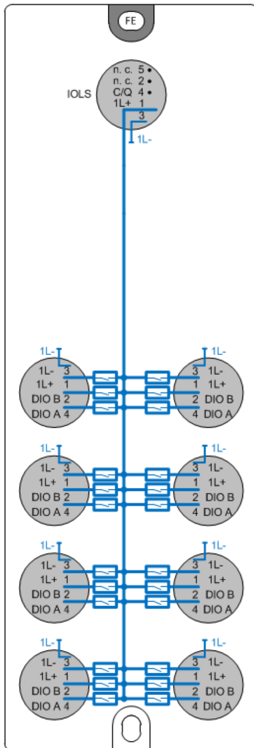
Abbildung 8: Prinzipschaltbild der Versorgung
