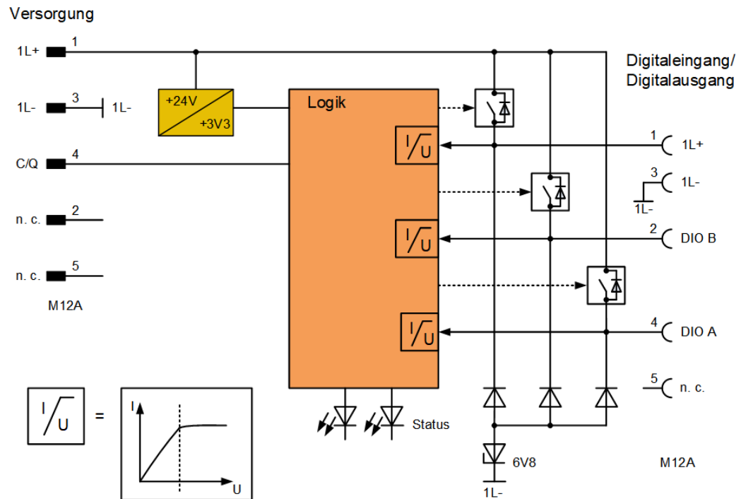
Abbildung 4: Schematisches Schaltbild je Port
