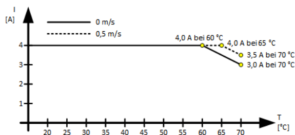
Abbildung 5: Derating 765-1703/200-000
