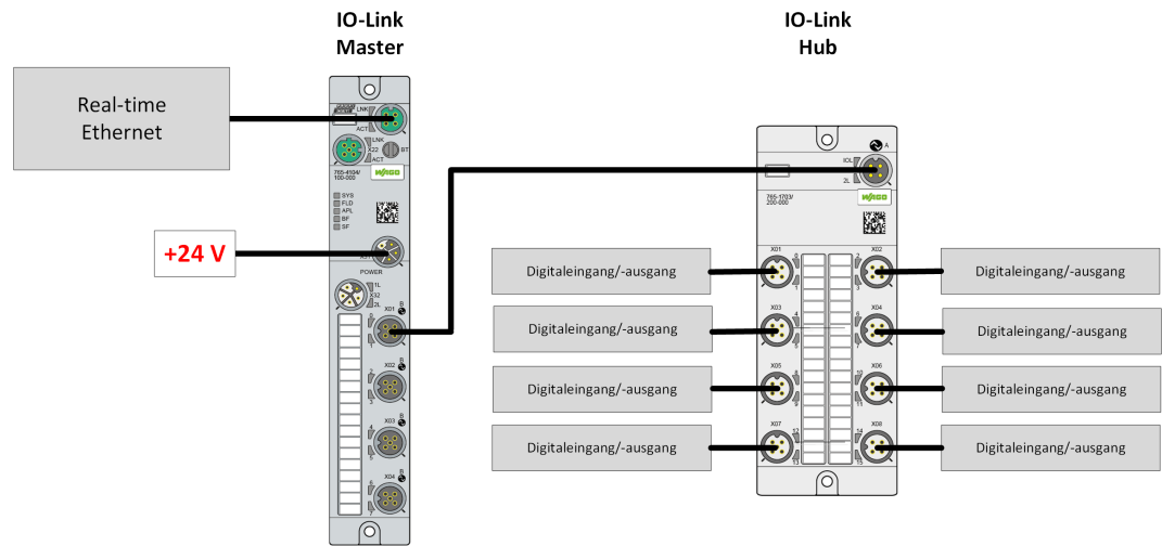
Abbildung 7: Anschlussbeispiel eines IO-Link-Hubs 765-1703/200-000 an einen IO-Link-Master
