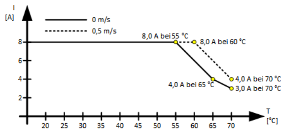
Abbildung 5: Derating 765-1706/200-000
