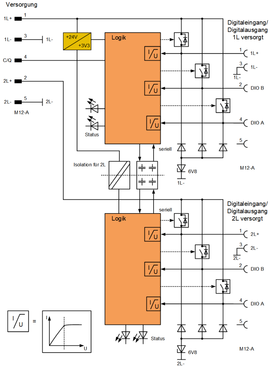
Abbildung 4: Schematisches Schaltbild je Port
