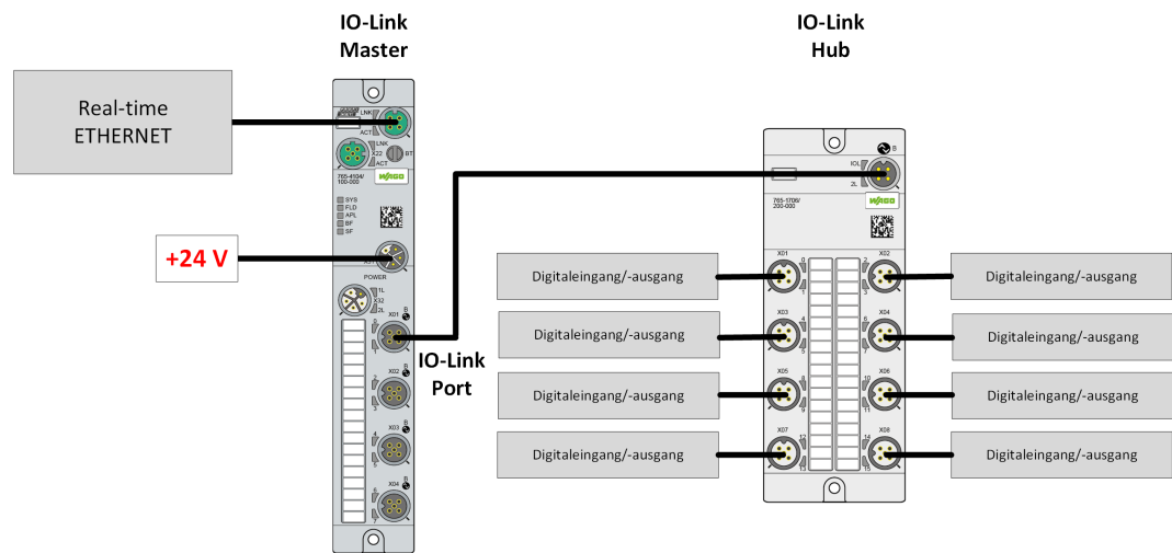
Abbildung 7: Anschlussbeispiel eines IO-Link-Hubs 765-1706/200-000 an einen IO-Link-Master
