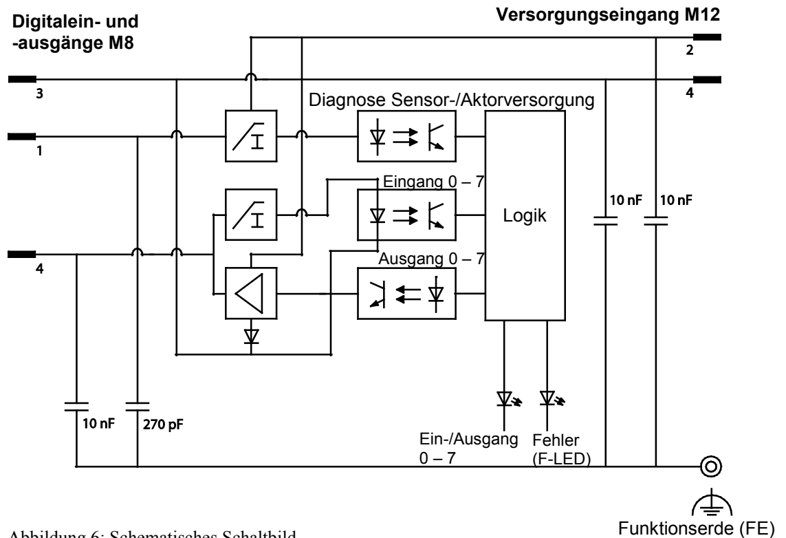
Abbildung 6: Schematisches Schaltbild
