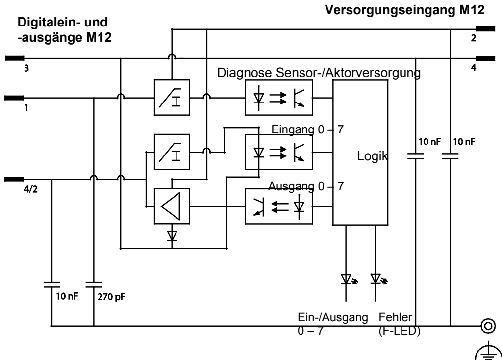
Abbildung 6: Schematisches Schaltbild
