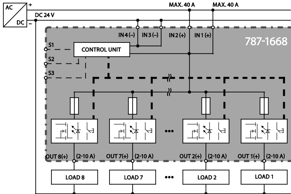
Figure 11: exemple de connexion
