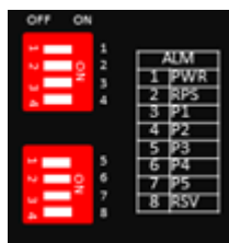
Fig. 6: Commutateurs DIP
