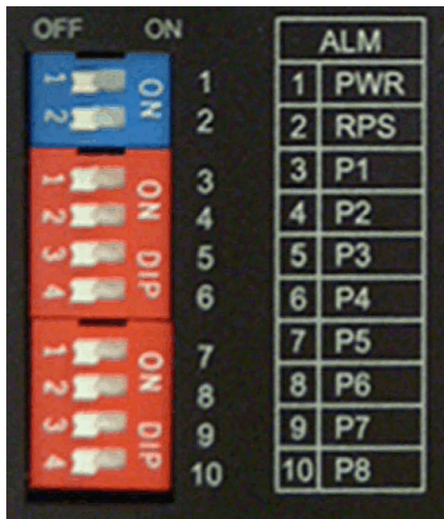
Fig. 6: Commutateurs DIP
