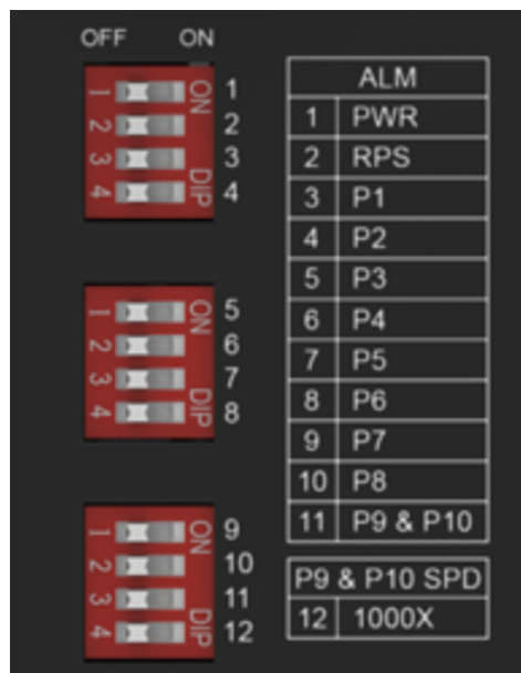
Fig. 6: Commutateurs DIP
