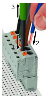
Fig. 10: Connexion de conducteur dans la Push-in CAGE CLAMP®
