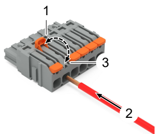
Fig. 14: Connexion de conducteur dans la Push-in CAGE CLAMP®
