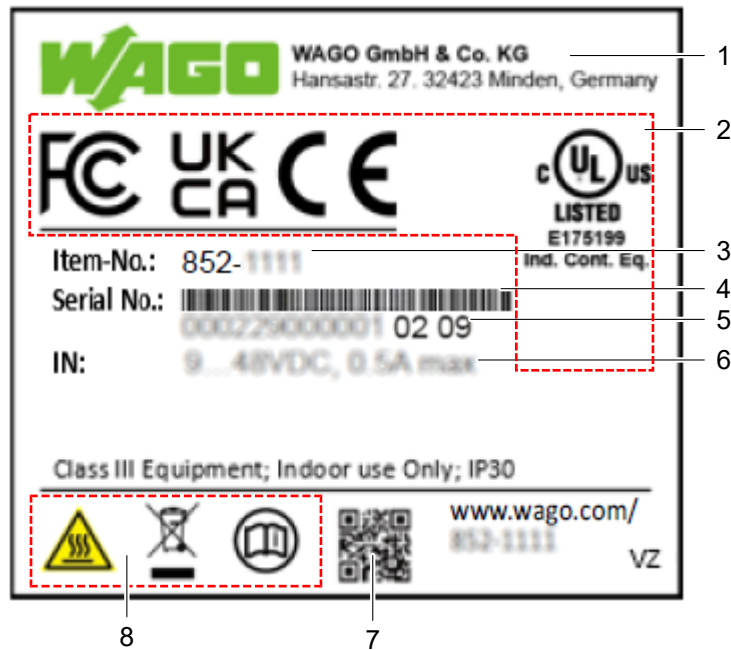
Fig. 3: Plaque signalétique (exemple)
