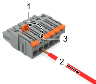
Fig. 15: Déconnexion des conducteurs de la Push-in CAGE CLAMP®
