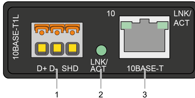
Fig. 1: Vue du bas
