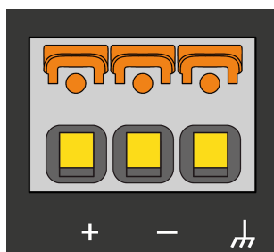
Fig. 4: Connexion d'alimentation
