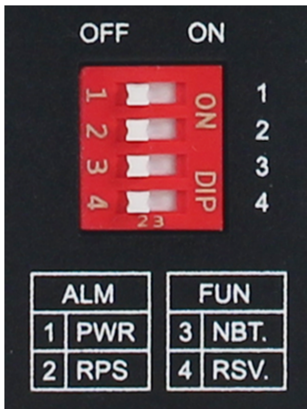
Fig. 6: Commutateurs DIP
