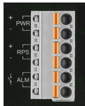
Fig. 3: Connexion d'alimentation (exemple)
