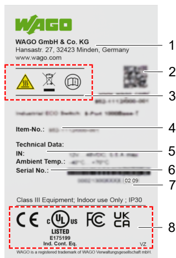
Abbildung 2: Typenschild (Beispiel)
