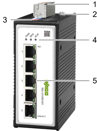
Abbildung 1: Frontansicht
